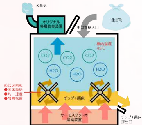
装置の断面イメージ
